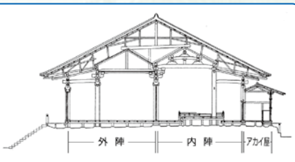
【當麻寺本堂(国宝)】断面図 内陣、外陣が一つの大屋根の中にあり、参詣礼拝空間が広くなった。大屋根を支える小屋組構造は古代、中世ではこのような自在な施工であった。アカイ屋とは闘伽井と書き、仏前に供える水を調えるところ。
